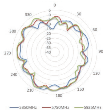
5350-5925 MHz
