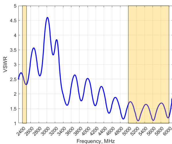
VSWR
